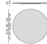
卓上回転台
